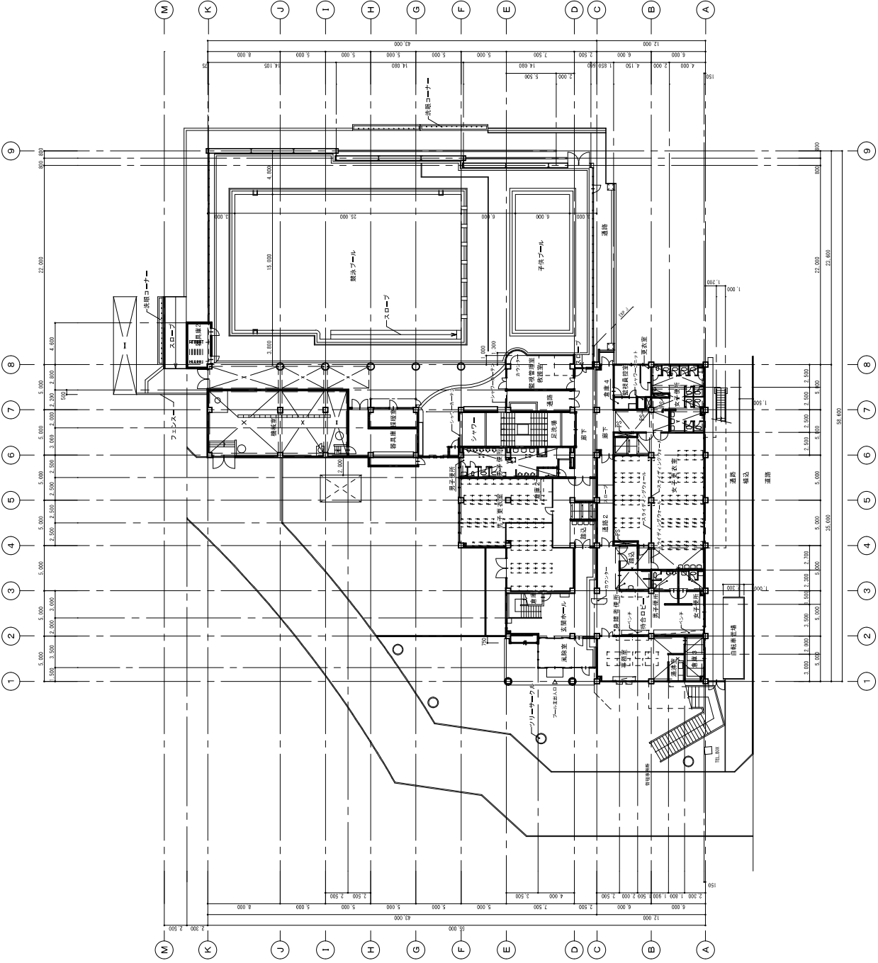
1階平面図 S=1/400
