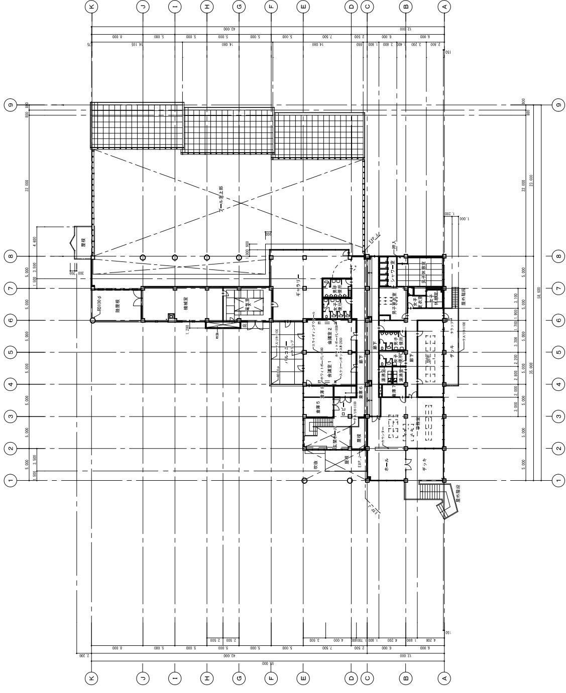
2階平面図 5=1/400
