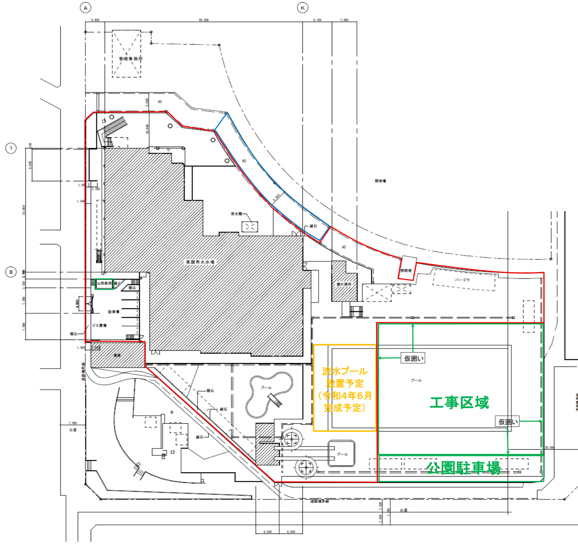
配置図 S=1/600
