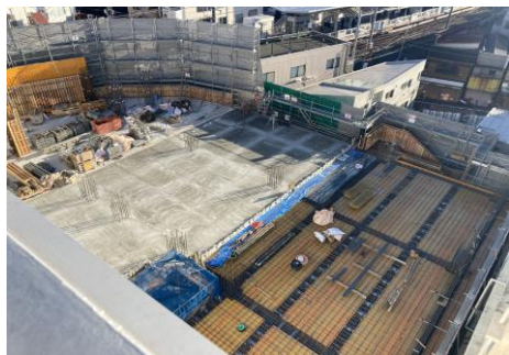
2階躯体工事
