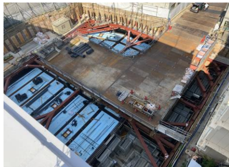
基礎躯体工事
