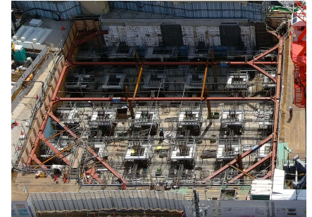
基礎工事
