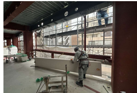
外装工事
