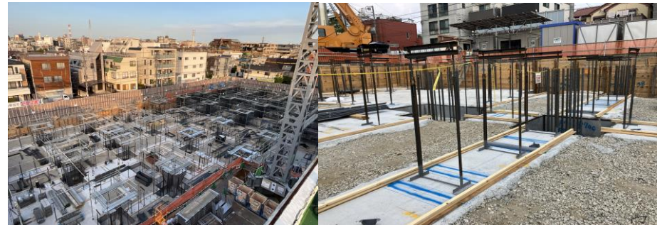
基礎工事
