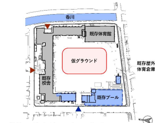
②特別教室棟・プール解体
