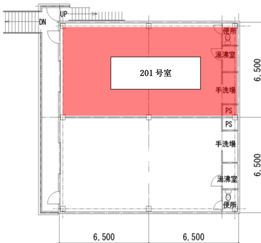
2階平面図
