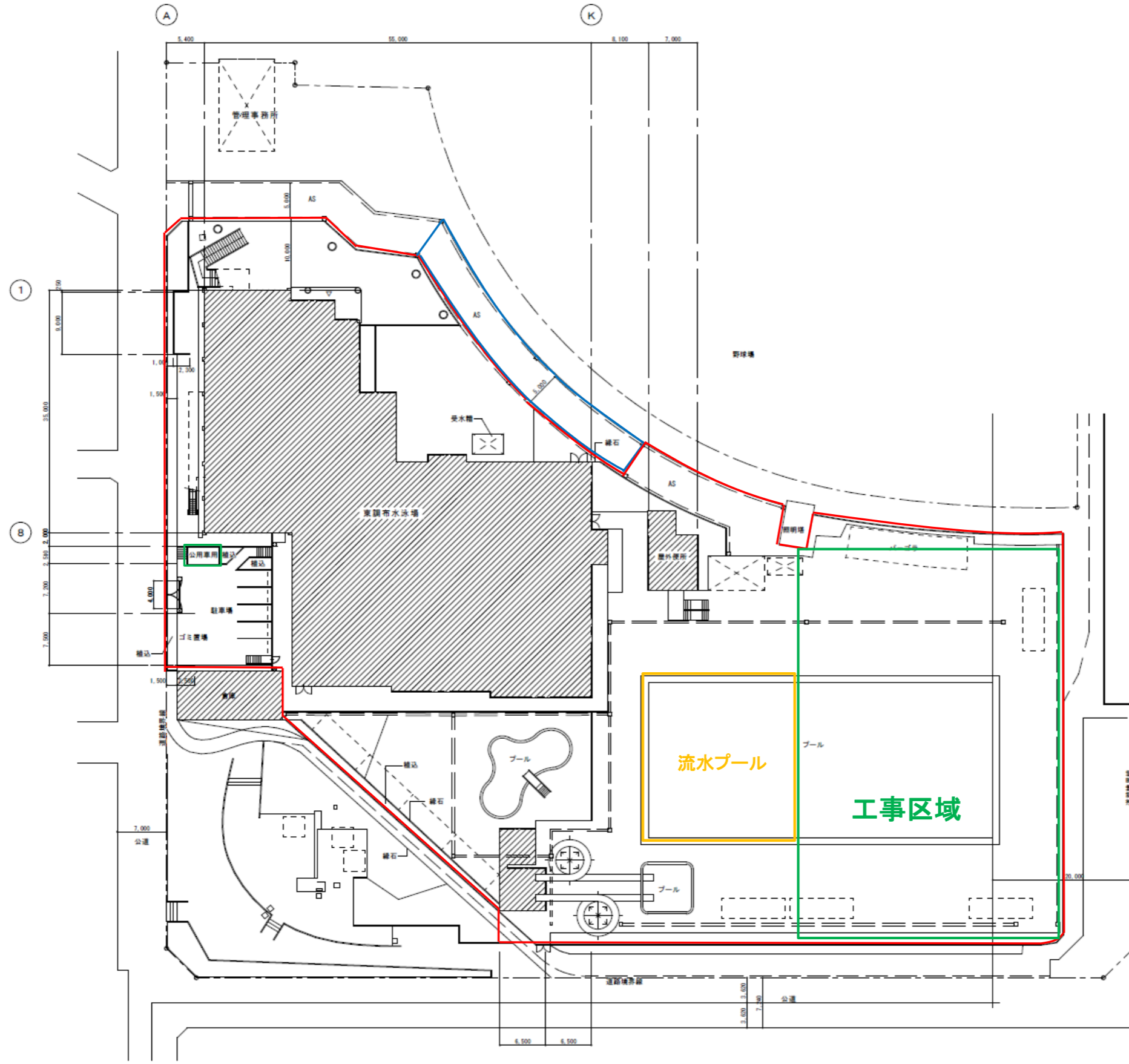
配置図 S=1/600
