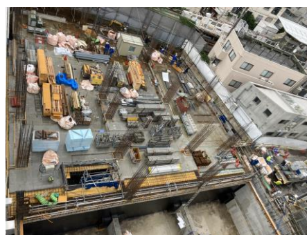
1階躯体工事
