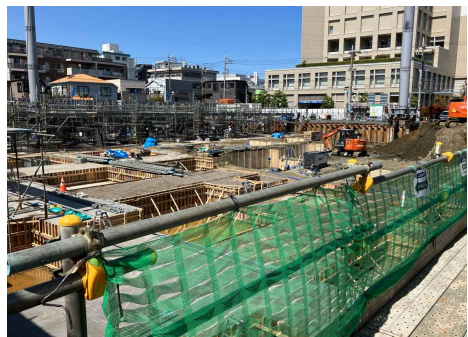
基礎工事
