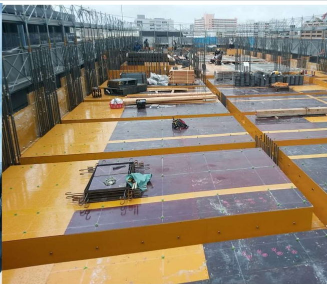
躯体工事 4階内部
