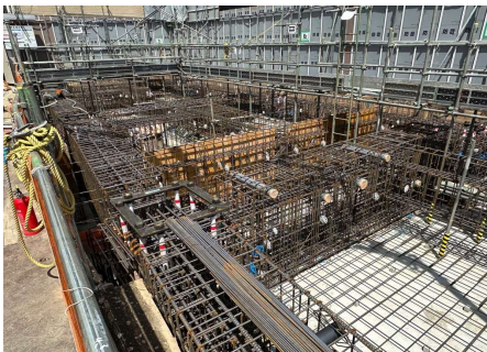
基礎工事
