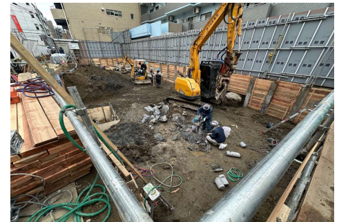
山留工事
