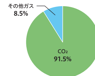
令和3年度温室効果ガス排出量のうち、CO 2 が占める割合
