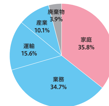
令和3年度CO 2 排出量（部門別割合）
