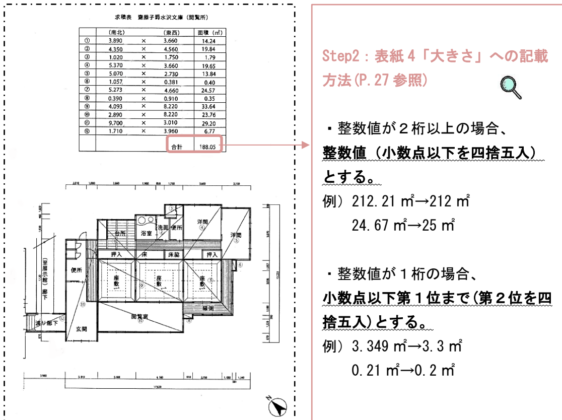
図1-10 求積図及び求積図の作成例
