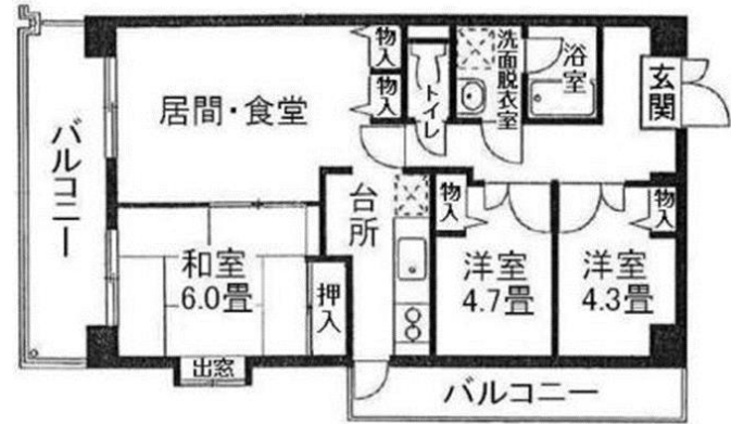
プラムハイツ大森西 Aタイプの主な間取り
